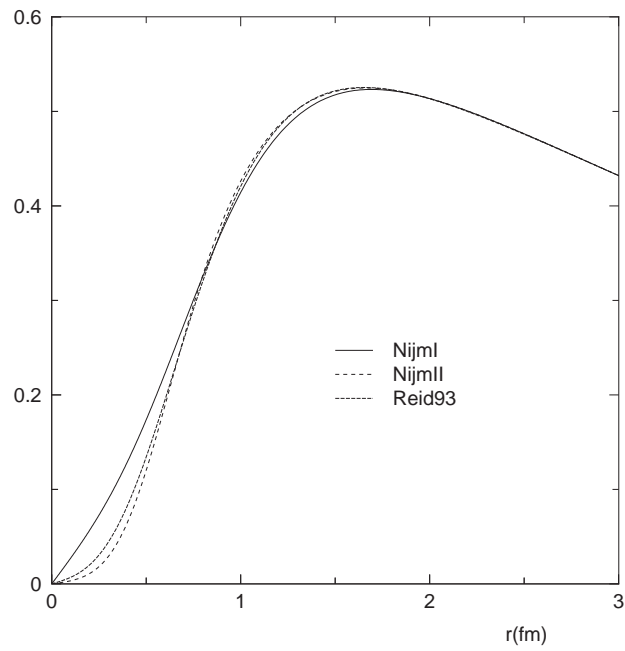
FIG. 3. The deuteron s -state wave function u(r) .
