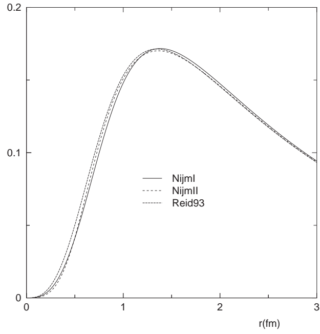
FIG. 2. The deuteron d -state wave function w(r) .
